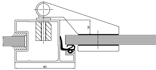
Przekrój słupka i poprzeczki górnej drzwi
