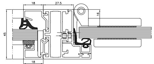
Przekrój słupka drzwi
